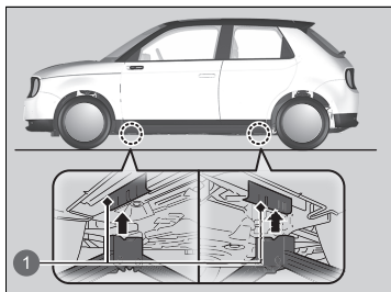
1 Zdvíhacie body
