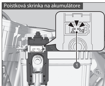
1 Vypálená
